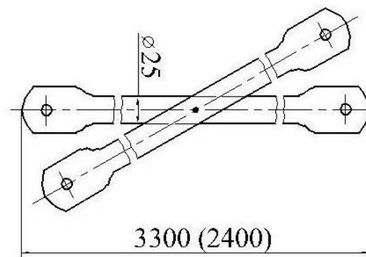
Ригель настила (7)
