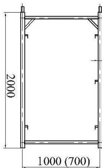
Рама без лестницы (1)
