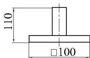
Опорная пята (5)
