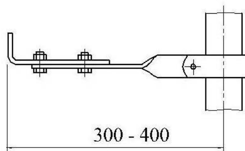
Кронштейн крепления (6)
