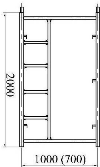
Рама с лестницей (2)
